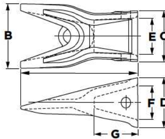
TYPE 15 - UT TWIN TIGER
