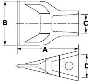
TYPE 14 - FLARE STANDARD
