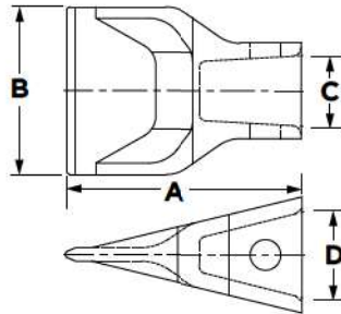
TYPE 14 - STANDARD FLARE
